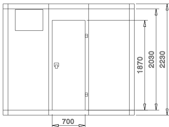
Boční
